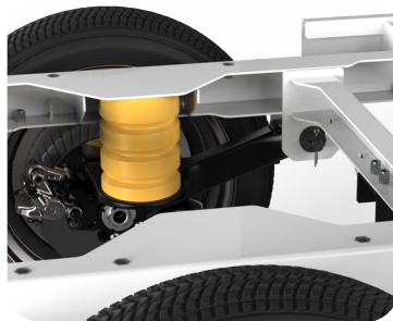
Vorderrad- und Hinterradfederung
